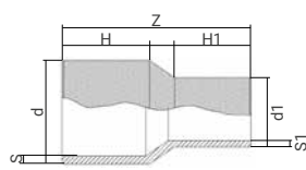
Diamètres 50 à 160 mm
