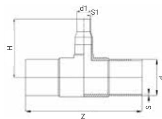
Diamètre 280 mm
