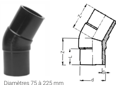
Diamètres 75 à 225 mm
