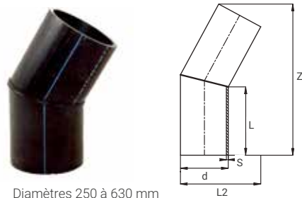
Diamètres 250 à 630 mm
