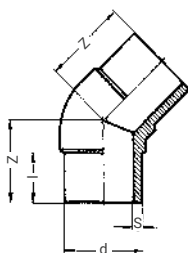
Diamètres 63 à 500 mm
