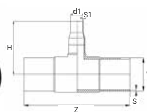
Diamètre 280 mm
