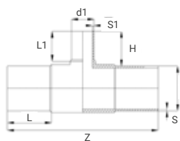
Diamètres 110 à 315 mm (sauf 280 mm)
